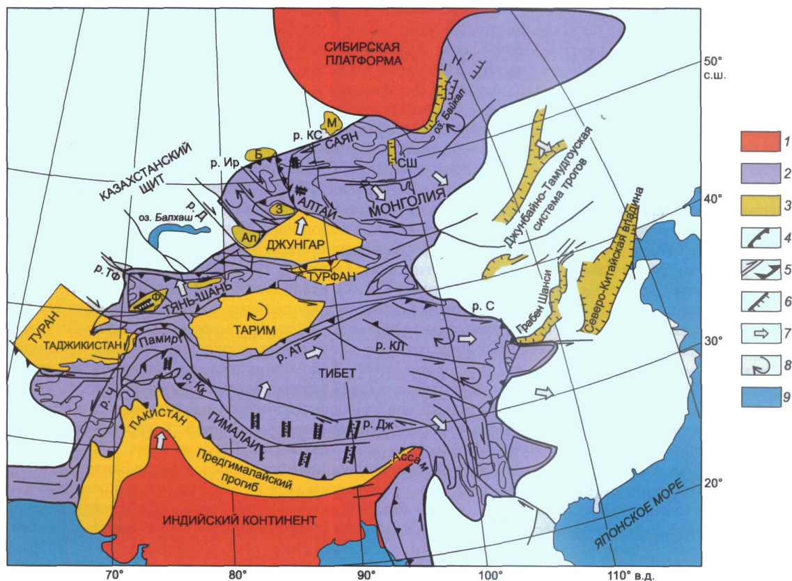
Рис. 1. Схема кайнозойских структур Центральной Азии, по [Dobretsov et al., 1996].
