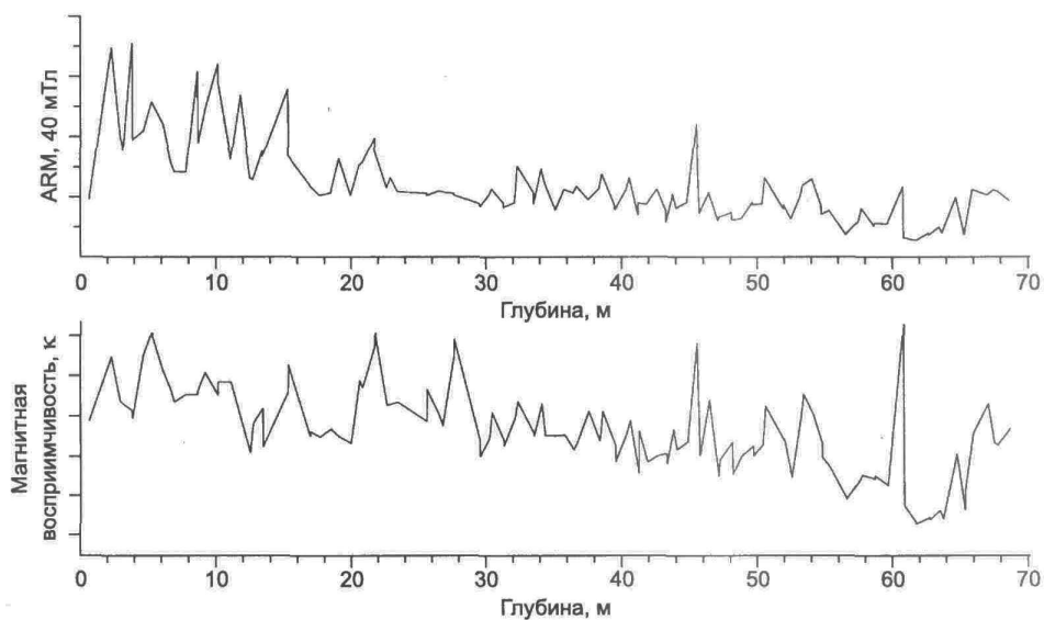
Рис. 4. Изменение магнитной восприимчивости и идеальной намагниченности в осадках верхней части скв. BDP-99.
