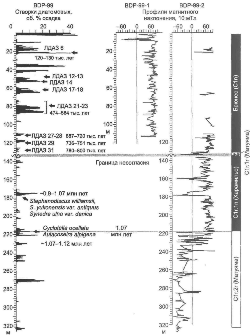
Рис. 3. Изменение наклонения NRM осадков скв. BDP-99 с глубиной (наст. работа) и сопоставление с данными диатомовой стратиграфии [Khursevich et al., 2005].
