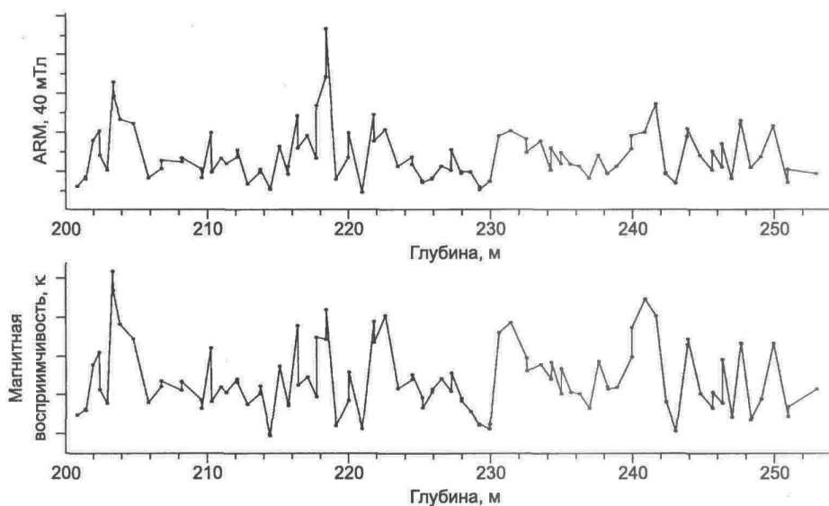
Рис. 5. Изменение магнитной восприимчивости и идеальной намагниченности в осадках скв. BDP-99 в период инверсии Харамильо—Матуйама.
