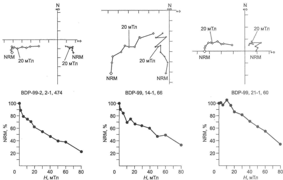
Рис. 2. Примеры детального размагничивания отдельных образцов.
