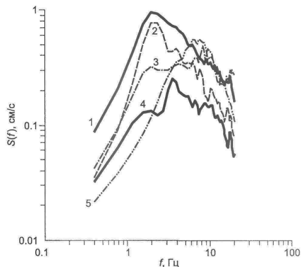
Рис. 4. Средние спектры ускорений землетрясений с M = 5.0—5.4 , имеющих разные подвижки в очаге, и афтершока Култукского землетрясения.
