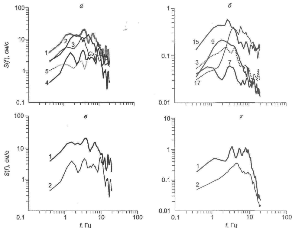
Рис. 3. Спектры ускорений Култукского землетрясения, зарегистрированного различными сейсмостанциями ( а ), спектры ускорений различных землетрясений с M = 5.0 — 5.4 , зарегистрированных на одной сейсмостанции ГС СО РАН — Монды ( б ), примеры спектров ускорений Култукского ( в ) и Южно-Байкальского ( г ) землетрясений на сейсмостанциях, расположенных параллельно тензору сейсмического момента (1) и поперек ему (2).
