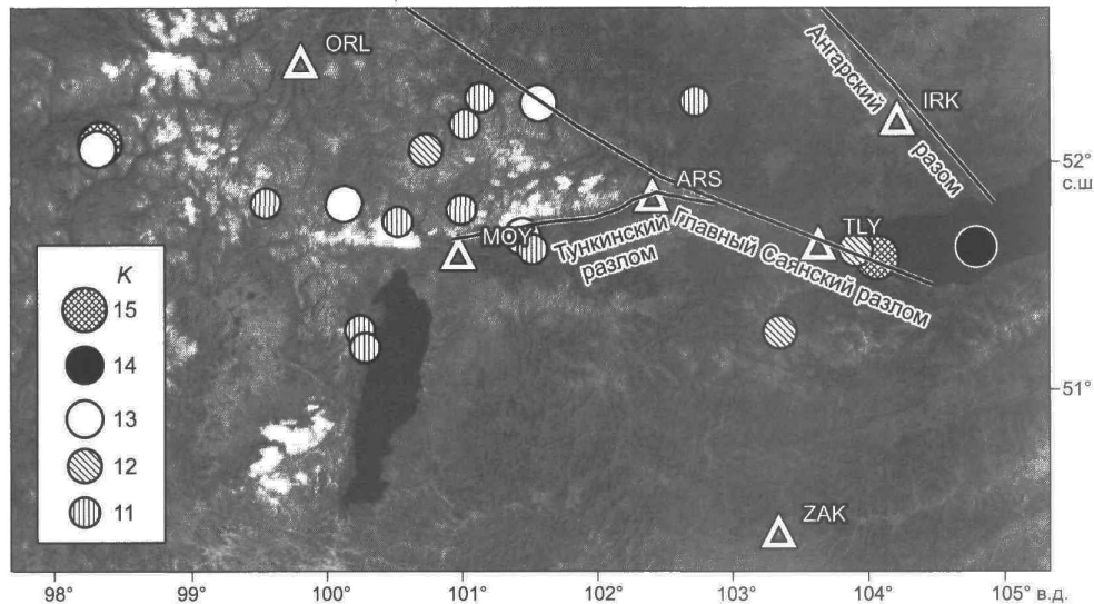
Рис. 1. Карта эпицентров землетрясений юго-западной части Байкальской рифтовой зоны за 1999—2009 гг., M > 4.0 .
