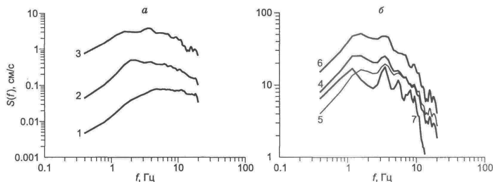
Рис. 5. Средние спектры ускорений землетрясений разных магнитуд юго-западной части Байкальской рифтовой зоны (а) и расчетные спектры землетрясений для M = 7.5 (б).
