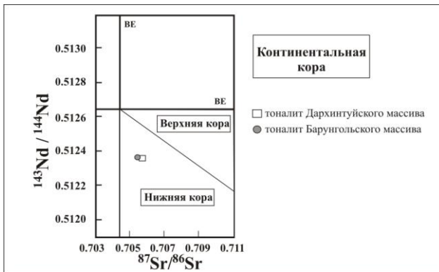
Рис. 8. Sr-Nd изотопные значения континентальной коры [Wilson M., 2003].
