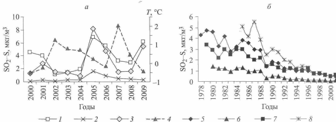
Рис. 1. Динамика среднегодовых концентраций SO 2 на станциях мониторинга Юго-Восточной Сибири (а) и Северной Европы (б).
