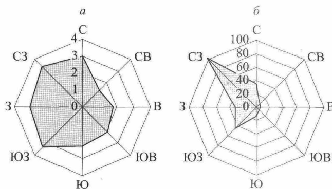
Рис. 3. Средние концентрации \text{SO}_2 ( \text{мкг}/\text{м}^3 ) на ст. Листвянка при разных направлениях ветров. а — лето; б — зима.
